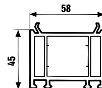
Blendrahmenverbreiterung 4,5 cm
