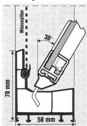
Flügel in Kippstellung
