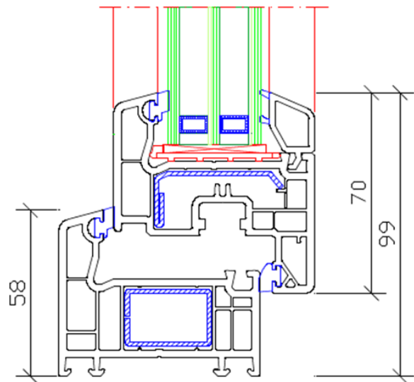
Schnitt ZO DKW Thermo Plus
