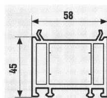
Blendrahmenverbreiterung 4,5 cm
