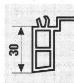
Fensterbankanschlußprofil 3 cm
