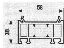
Blendrahmenverbreiterung 3 cm
